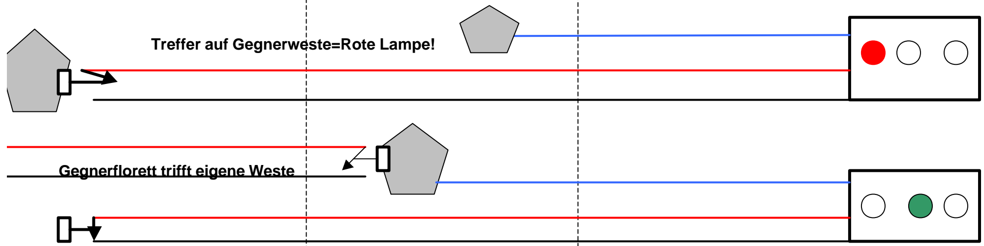
Florettfechten, Stromkreis-Schema, Blatt 2
